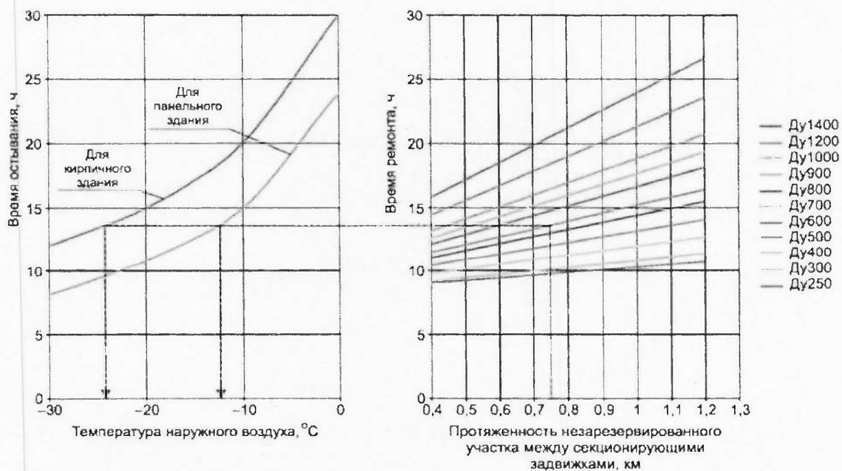
Рисунок 3 – Номограмма для определения периодов остывания для подъездов и лестничных клеток жилых зданий со снижением температуры с +15 до +3^{\circ}\text{C}
